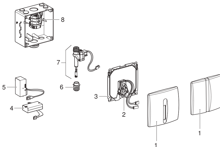
Илустрација 1: Geberit контролери на писоар со електронско пуштање вода, мрежна или батериска работа, Basic
