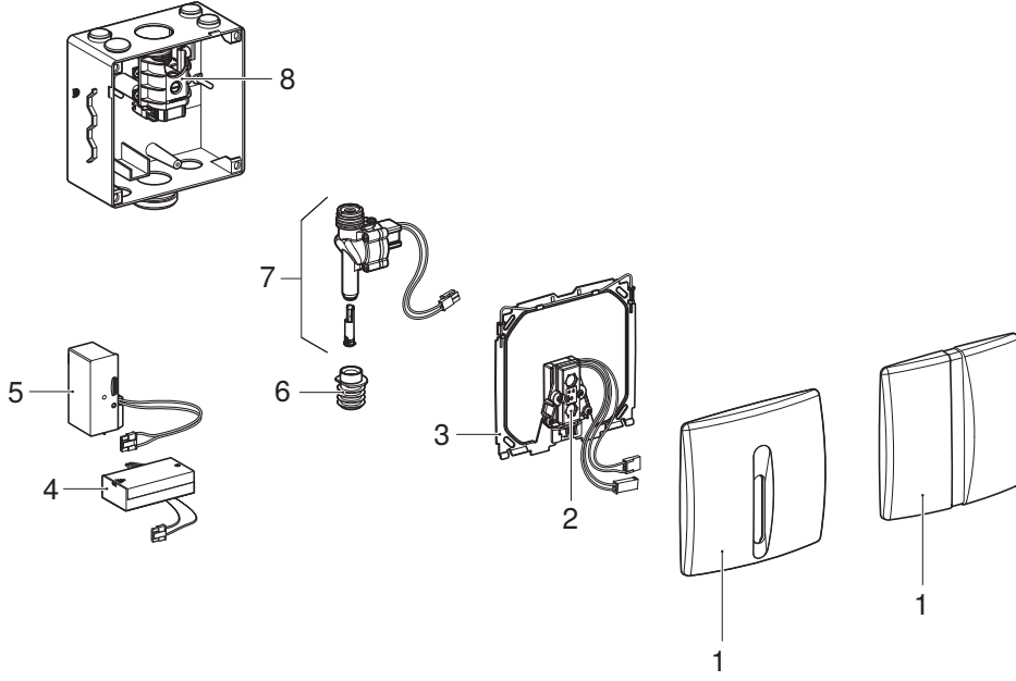
الشكل 1: أنظمة التحكم في مبولة Geberit المزودة بنظام تفعيل إلكتروني للشطف ونظام تشغيل بالشبكة أو البطارية، Basic.
