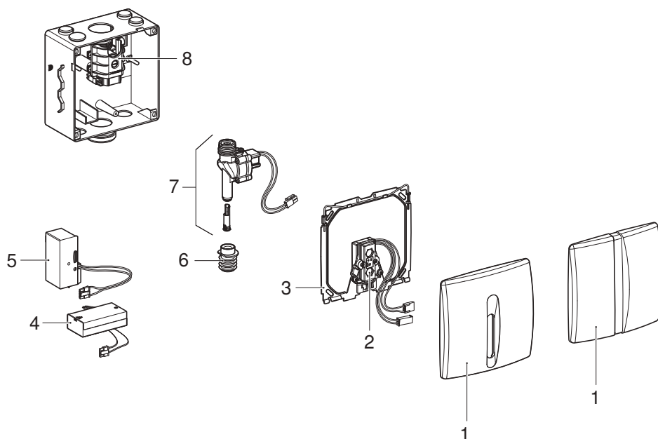
Ilustrimi 1: Njësitë e komandimit të pisuareve Geberit me aktivizim elektronik të shpëlarjes, me funksionim elektrik ose funksionim me bateri, Basic
