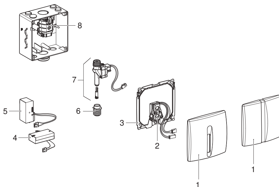
Rysunek 1: Zawory spłukujące do pisuarów Geberit z elektronicznym uruchamianiem spłukiwania, zasilanie sieciowe lub bateryjne, wersja Basic
