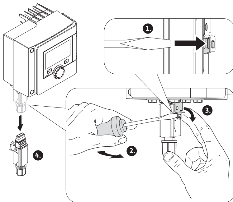
Fig. 30: Wilo-Connector demontieren
