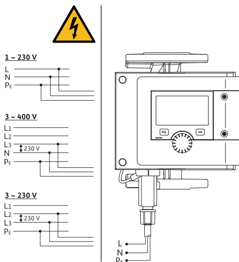
Fig. 23: Anschlussmöglichkeiten
