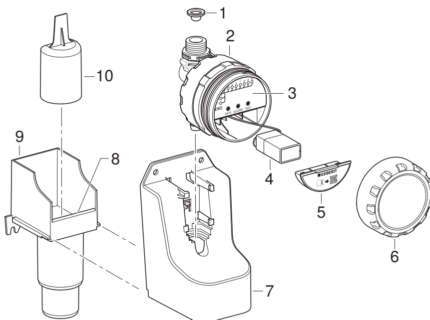
Ilustrimi 1: Qarkulluesi higjienik Geberit HS01
