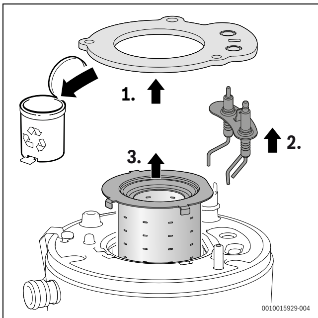
Bild 22 Brenner herausnehmen
