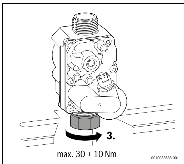
Bild 42 Anzugsdrehmoment beachten
