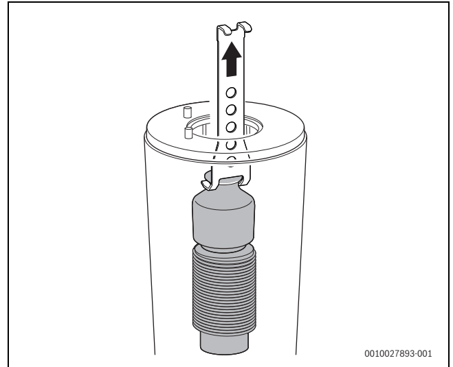
Bild 23 Oberen Verdrängungskörper herausnehmen
