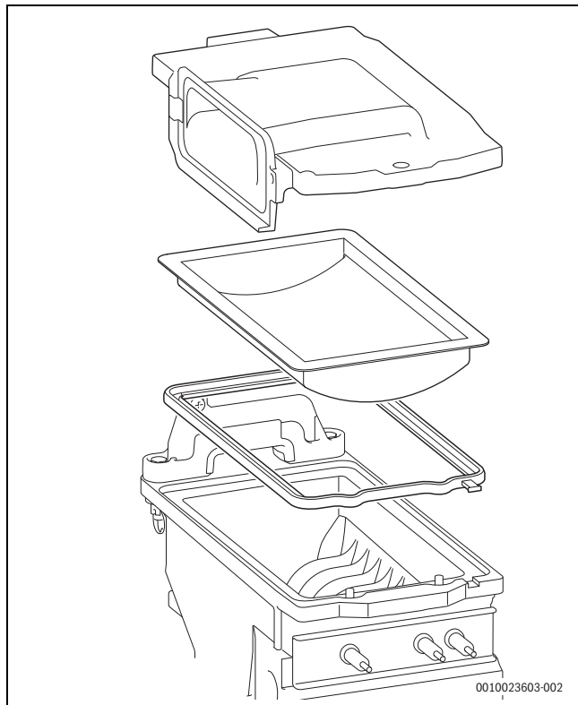
Bild 16 Brenner
