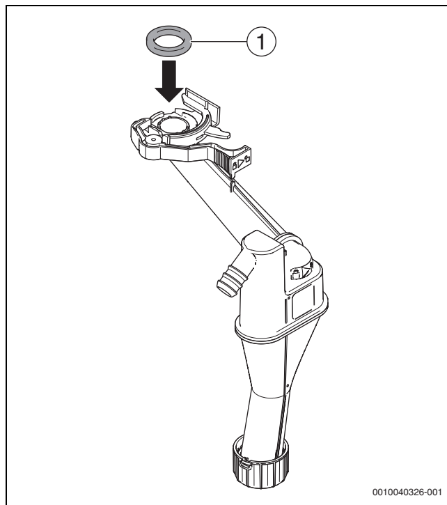
Bild 23 Neue Dichtung am Kondensatsiphon einsetzen
