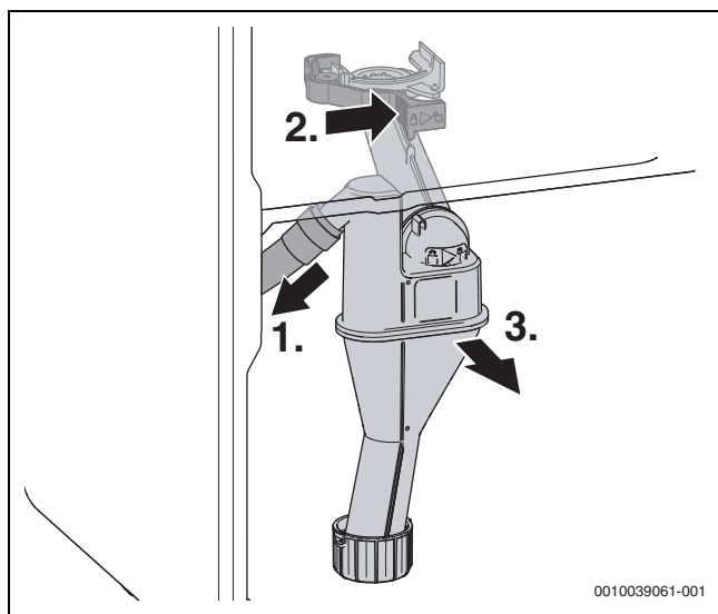
Bild 21 Kondensatsiphon ausbauen
