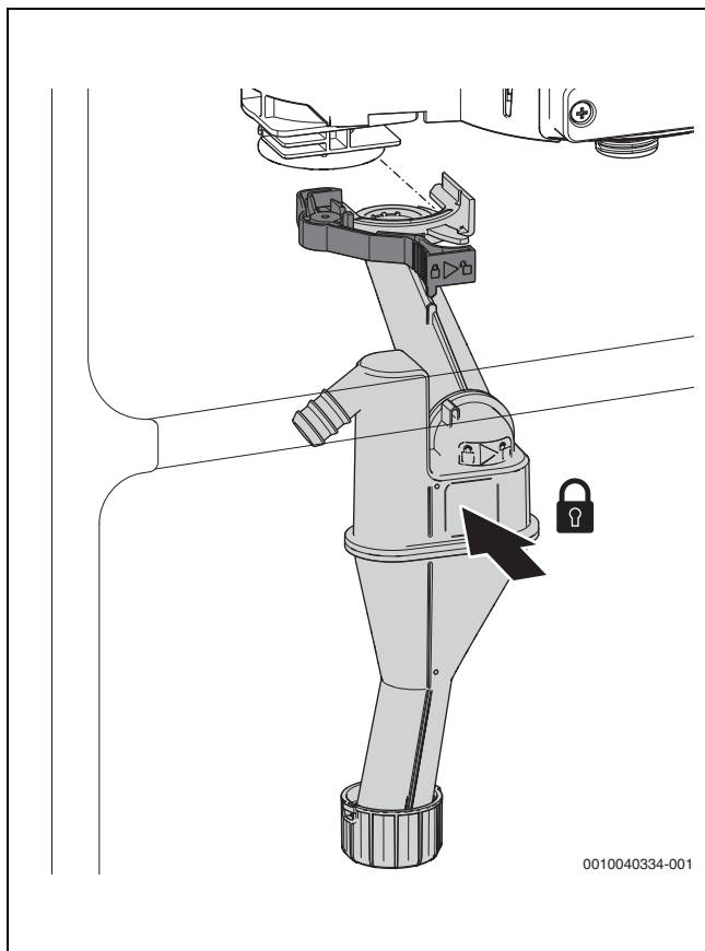
Bild 25 Kondensatsiphon einsetzen
