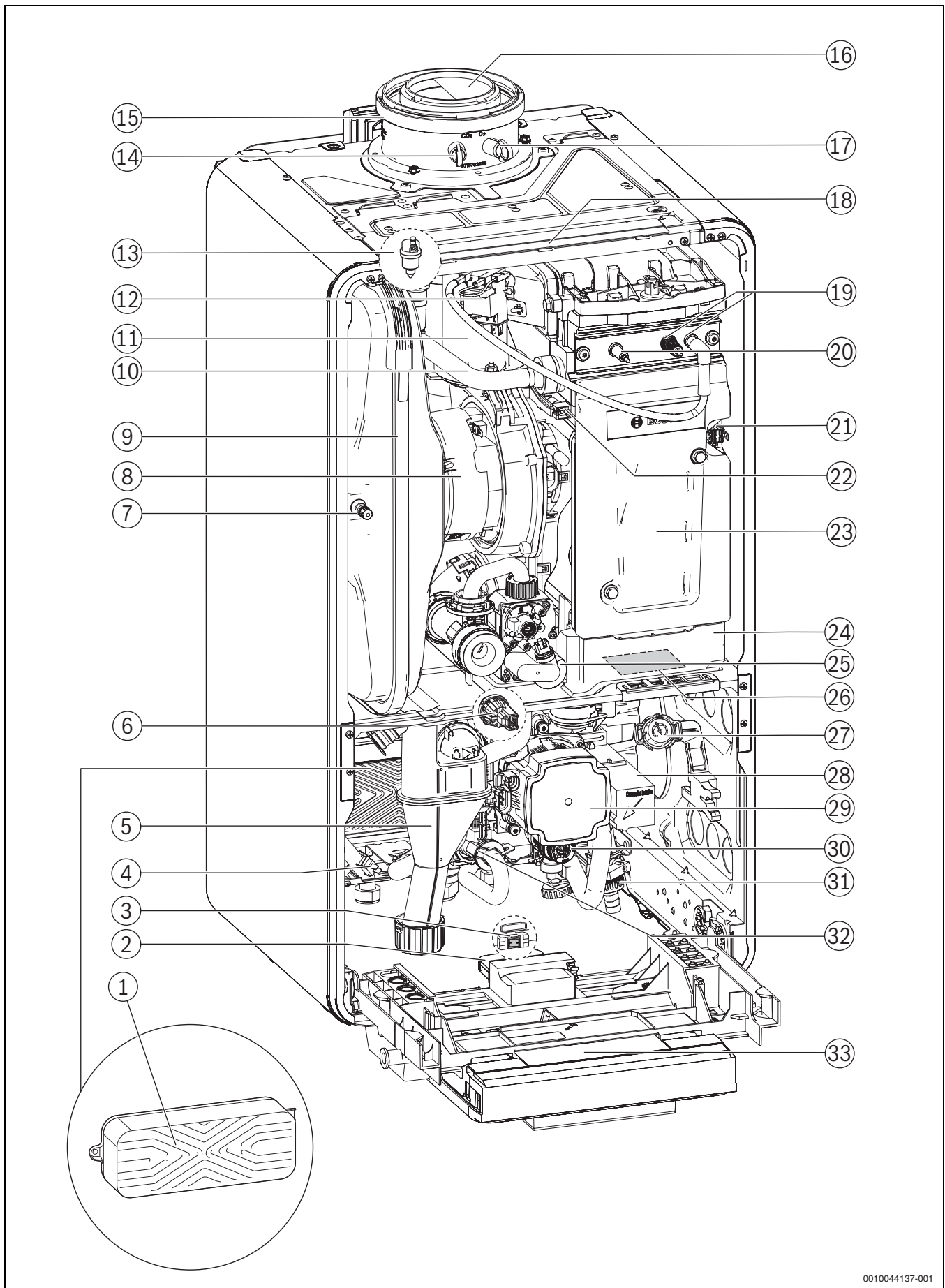
Bild 3 Produktübersicht Kombigerät
