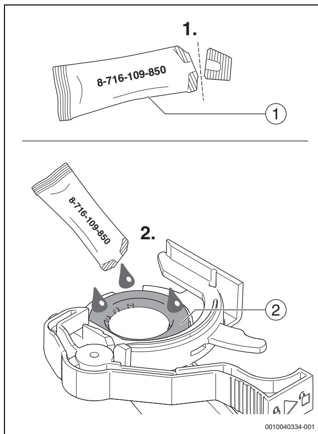
Bild 24 Dichtung fetten
