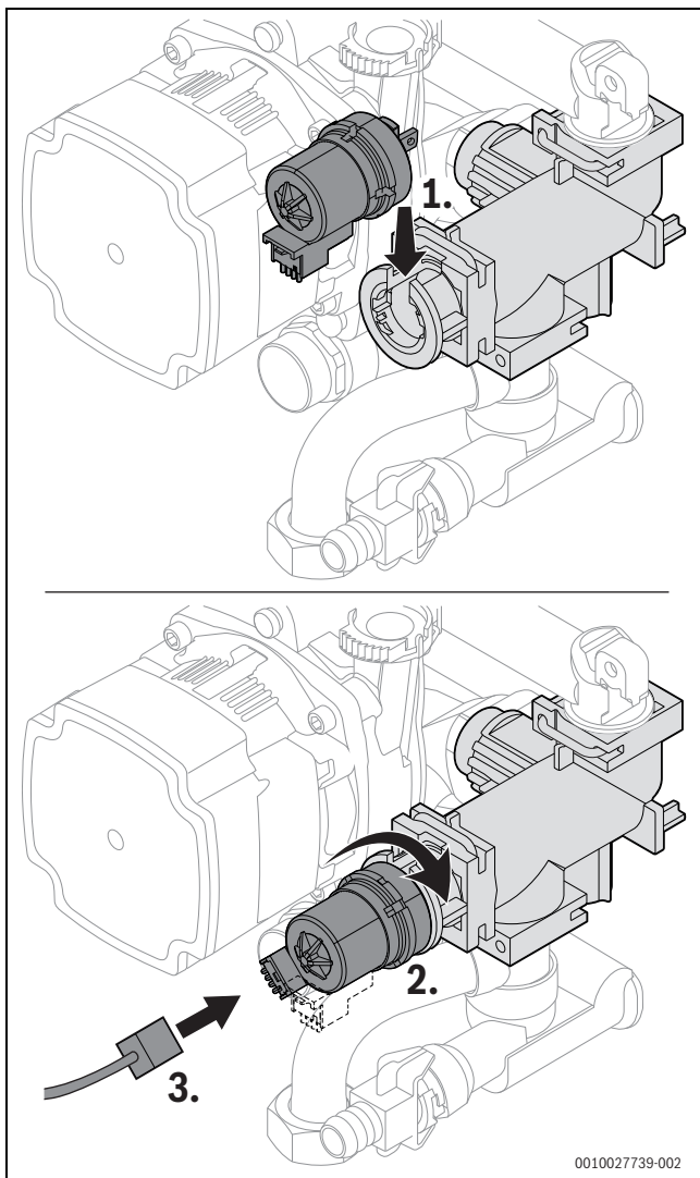
Bild 27 Motor am 3-Wege-Ventil einbauen (Variante ohne Schrauben)
