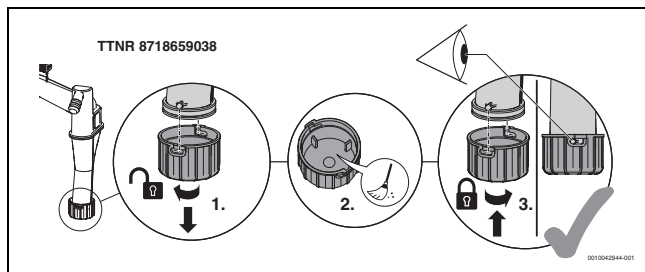
Bild 22 Schmutzfänger reinigen
