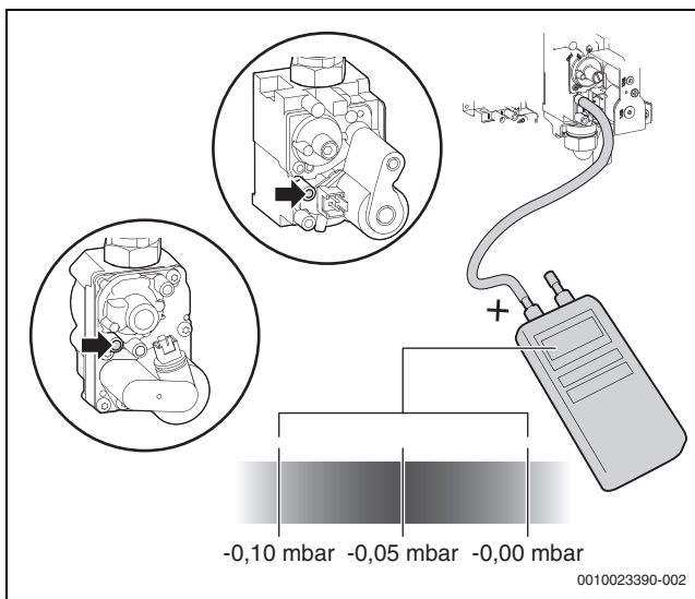
Bild 9 Differenzdruck messen
