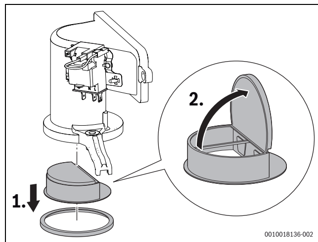
Bild 19 Rückschlagklappe in der Mischeinrichtung
