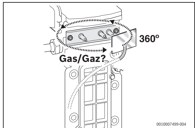
Bild 14 Dichtheit prüfen
