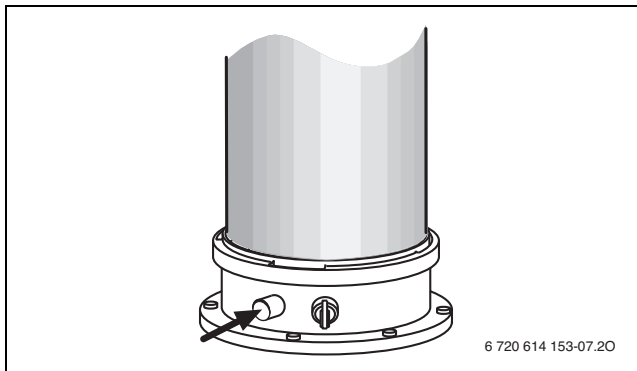
Bild 8 Abgasmessstutzen
