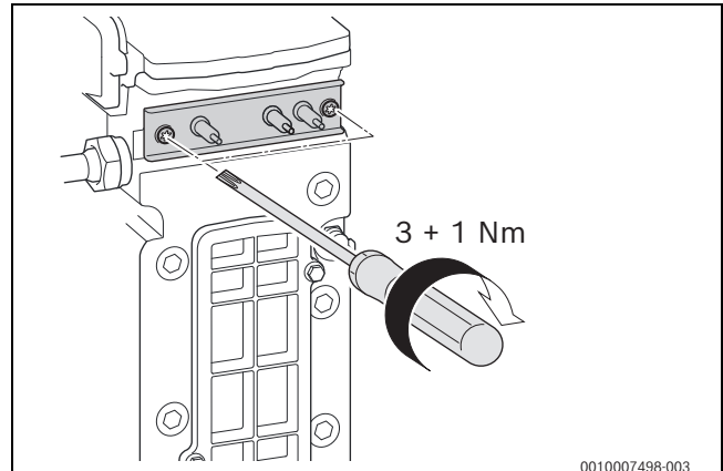
Bild 13 Elektroden-Set montieren
