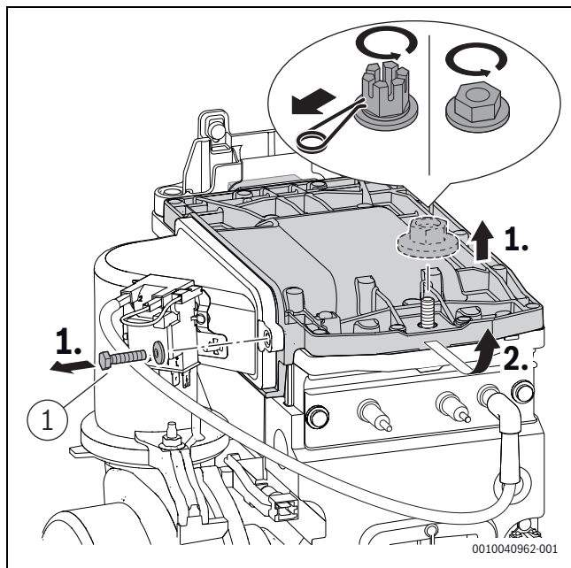
Bild 15 Brennerdeckel ausbauen
