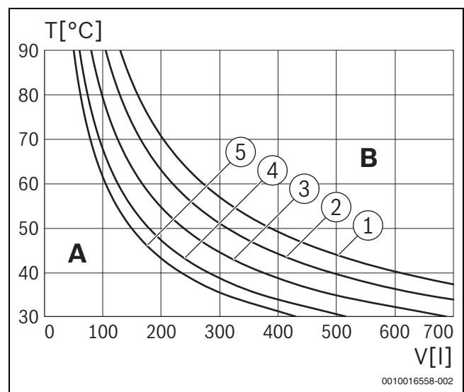
Bild 20 Kennlinien des Ausdehnungsgefäßes
