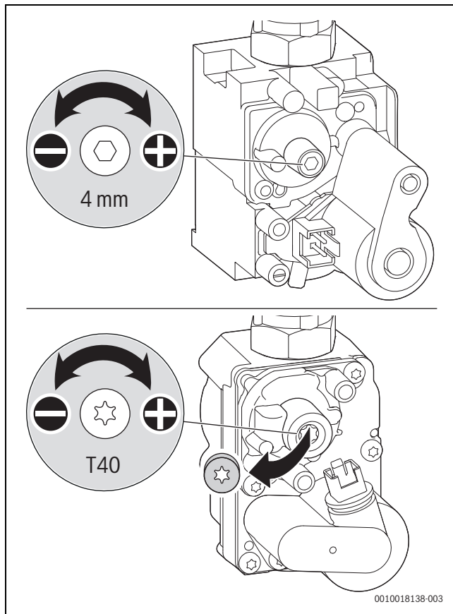
Bild 10 CO 2 - oder O 2 -Gehalt einstellen
