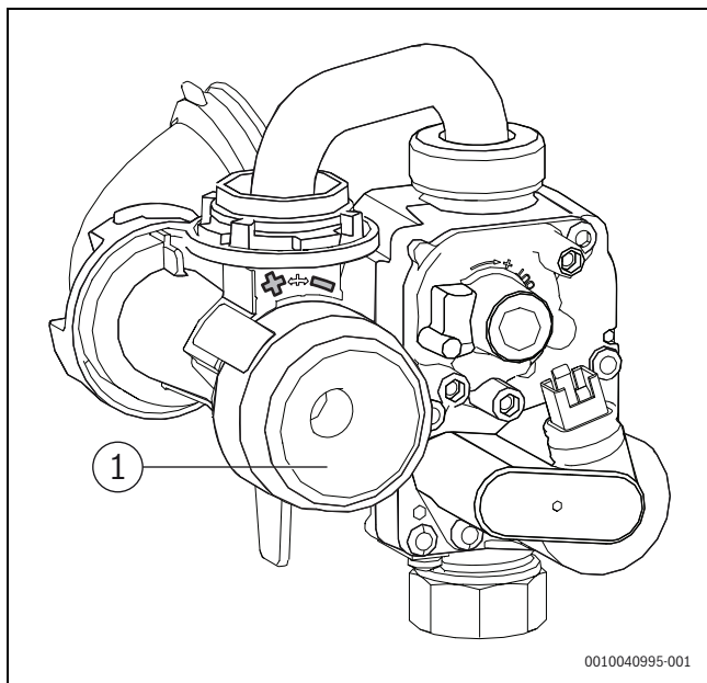
Bild 7 Gas-Luft-Verhältnis einstellen
