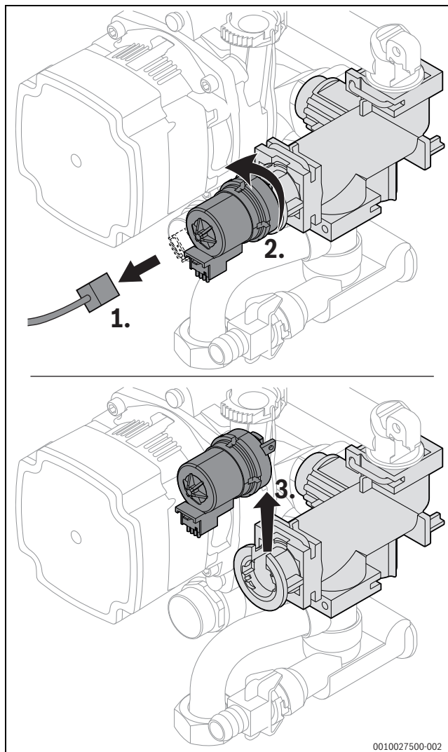
Bild 26 Motor am 3-Wege-Ventil ausbauen (Variante ohne Schrauben)
