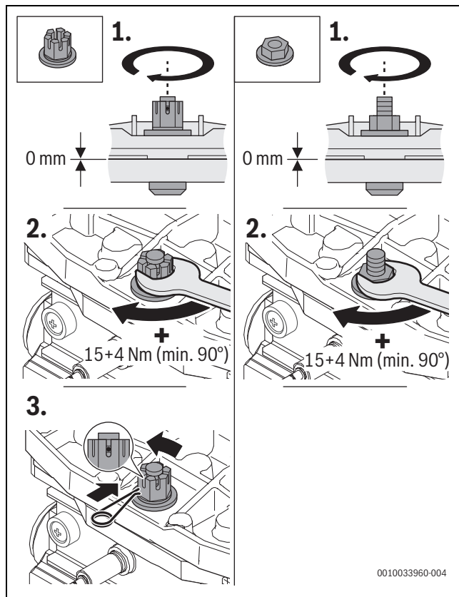
Bild 17 Mutter am Brennerdeckel festziehen
