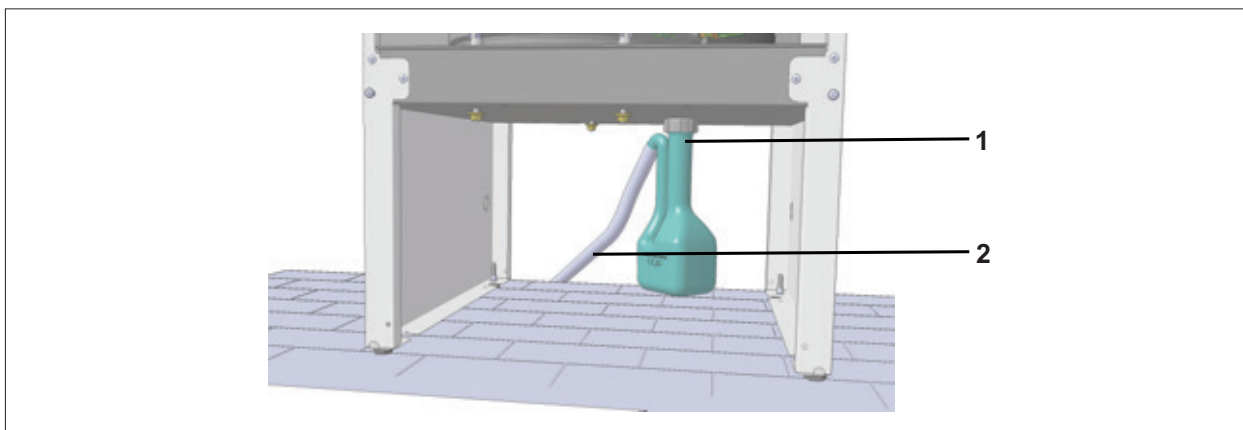
Abb. 4.12 Siphon demontieren
