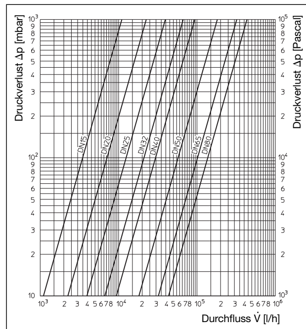
Durchflussdiagramm
