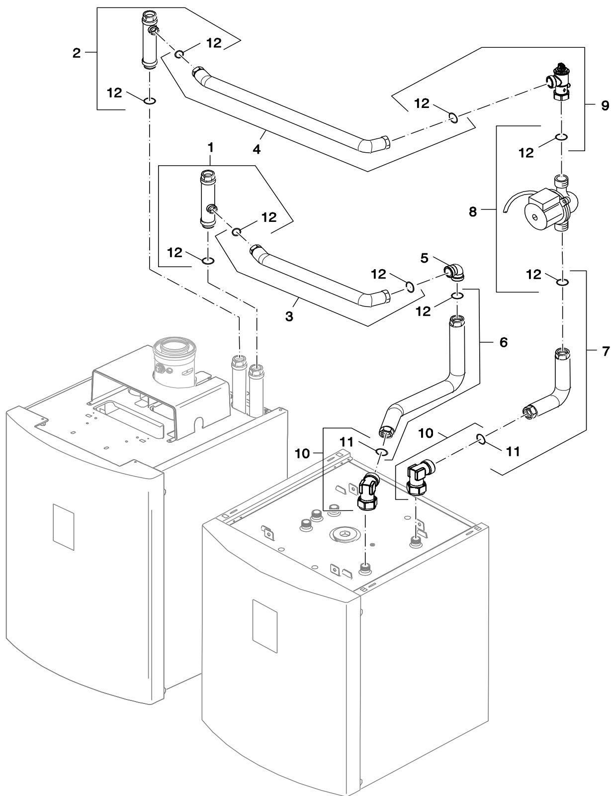
8738890515.aa.RS-Anschluss-Set Speicher nebeneinander
