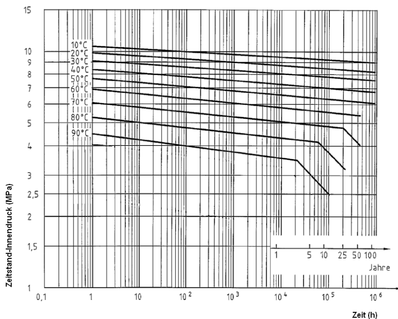
Zeitstand-Innendruckfestigkeit Roth Systemheizröhr
