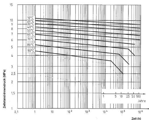
Zeitstand-Innendruckfestigkeit Roth Systemheizrohr X-PERT S5+
