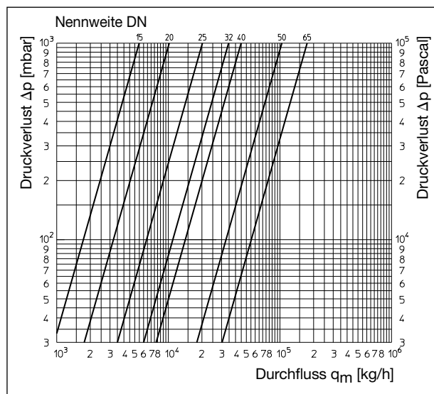
Durchflussdiagramm
