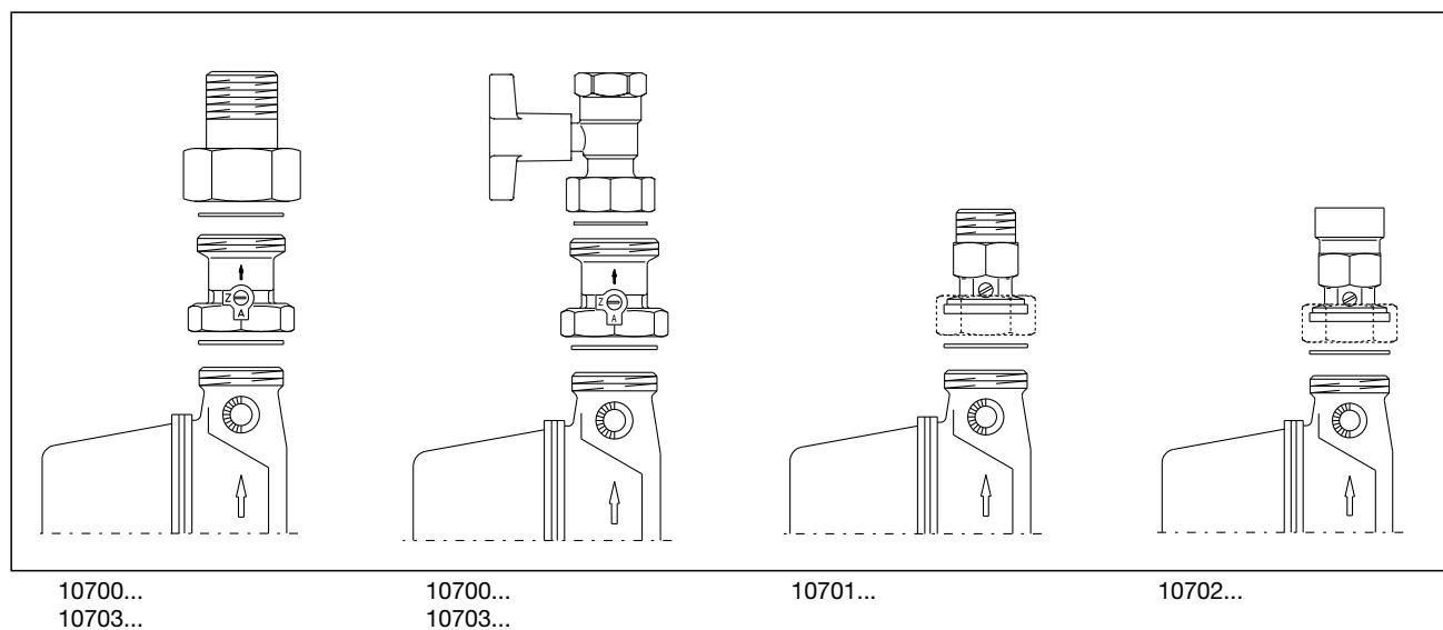
Einbaubeispiele
