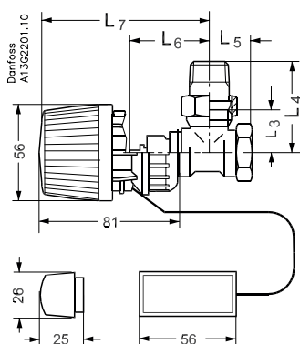
Element mit Fernfühler. Gehäuse in Eckausführung.
