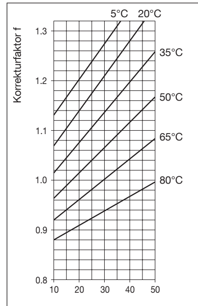
Gewichtsanteil Propylenglykol [%]
