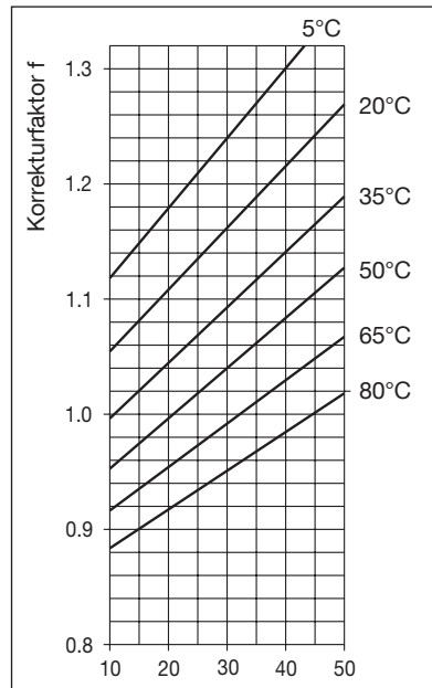
Gewichtsanteil Aethylenglykol [%]
