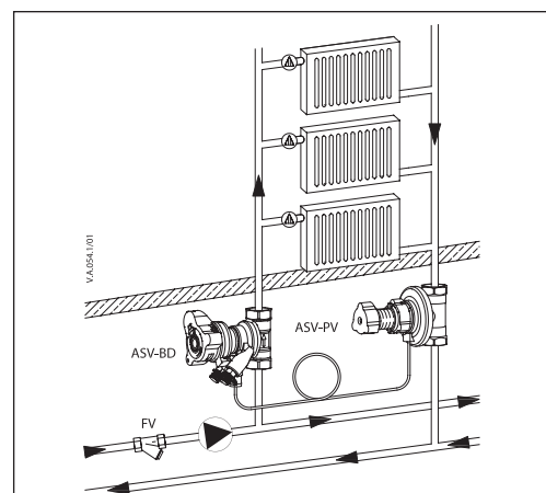
Abb. 3 ASV im vertikalen Strang/typische Heizkörperheizungsanwendung (allgemeines Beispiel)
