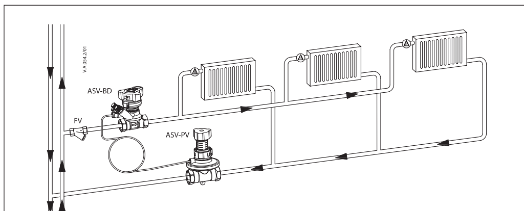
Abb. 4 ASV im horizontalen Strang/typische Heizkörperheizungsanwendung (allgemeines Beispiel)
