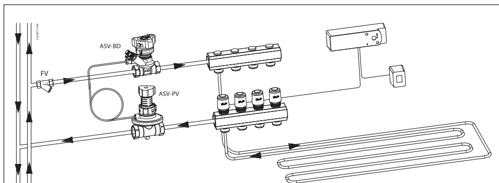
Abb. 5 ASV im Sammelrohr für eine Fußbodenheizung
