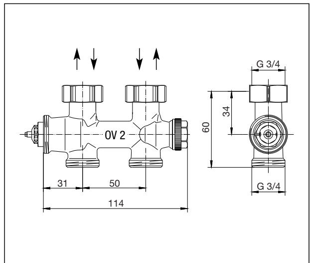
Durchgangsform
