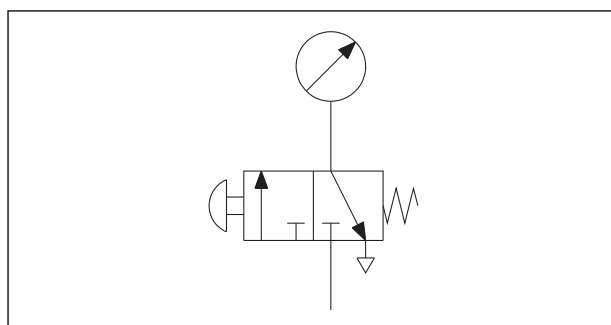
Schaltschema
