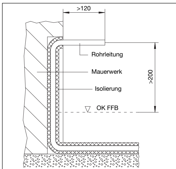
Schnitt, Heizkreisanschluss
