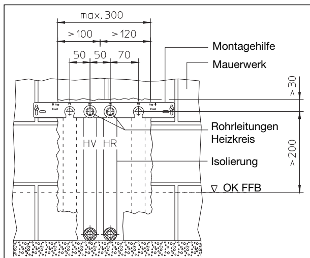
Wandansicht, Heizkreisanschluss
