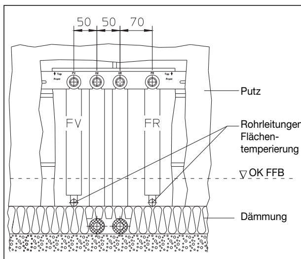
Wandansicht, Flächentemperierung
