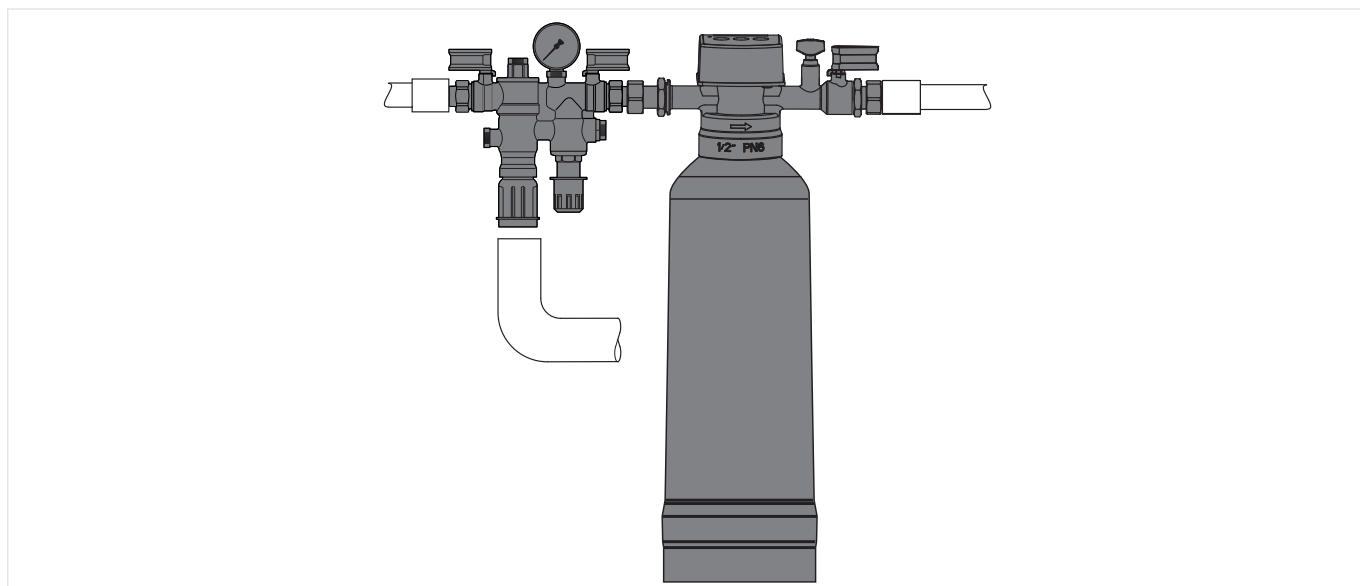
Abb. 1 Beispiel für den standardmäßigen Einbau der Nachfüllkombination
