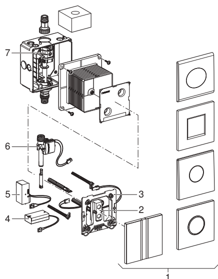
Ilustrimi 1: Njësitë e komandimit të pisuareve Geberit me aktivizim elektronik të shpëlarjes, me funksionim elektrik ose me bateri
