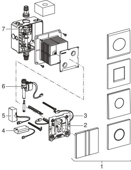
الشكل 1: أنظمة التحكم في مبدلة Geberit المزودة بنظام تفعيل إلكتروني للشطف ونظام تشغيل بالشبكة أو البطارية
