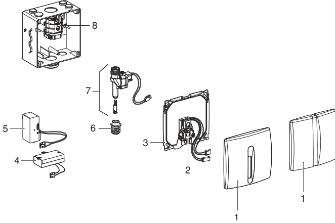
Şekil 1: Şebeke elektrliği ile veya pille çalışan, elektronik deşarj tetiklemeli Geberit Basic pisuvar deşarj kontrolleri
