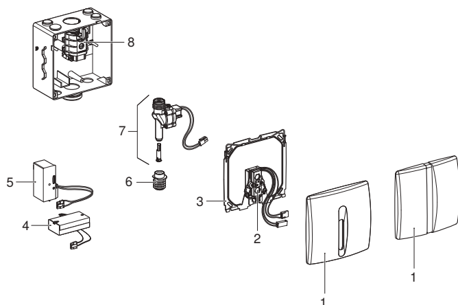
Mynd 1: Geberit þvagskálastýringar með rafrænni skolstjórnun sem eru tengdar við rafmagn eða ganga fyrir rafhlöðum, Basic
