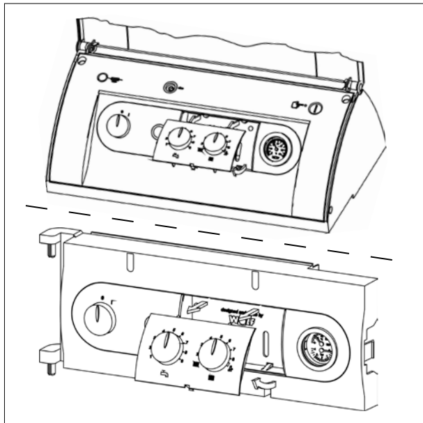
Abb. 4.8 Frontblende herausnehmen
