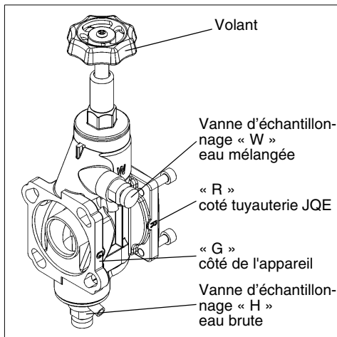
Fig. 1 : Montage JQX
