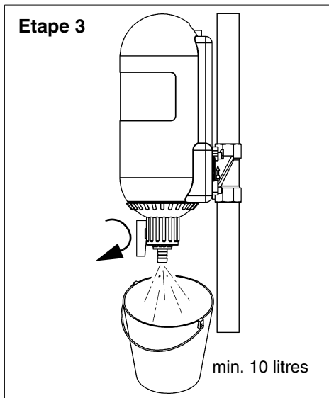
Fig. 8: Déclencher la performance du rétrolavage en ouvrant le robinet à boisseau sphérique. Un réservoir collecteur / seau avec une capacité de minimum 10 litres doit être disponible. Attention EAU CHAUDE / Danger de brûlure !
