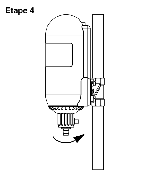
Fig. 9: Lorsque la performance du rétrolavage est terminée, fermer le robinet à boisseau sphérique et tourner en arrière. Ainsi l'appareil est de nouveau en position de service.
