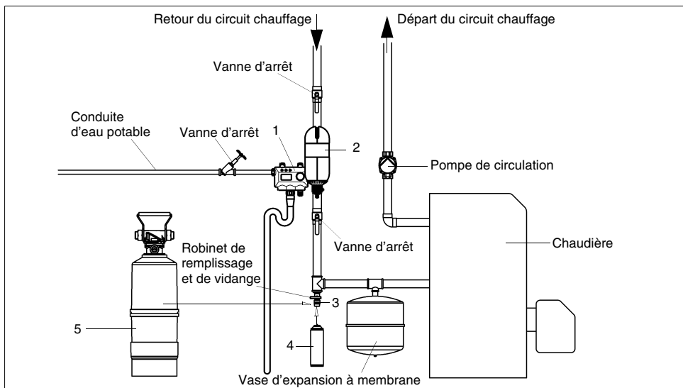
Abb. 2: Schéma JUDO HEIFI-TOP avec dispositif mobile de traitement de l'eau selon VDI 2035
