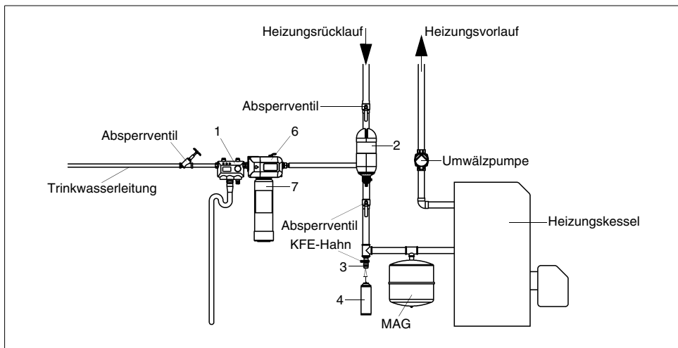
Abb. 3: Schema JUDO HEIFI-TOP mit stationärer Heizungswasseraufbereitung nach VDI 2035
