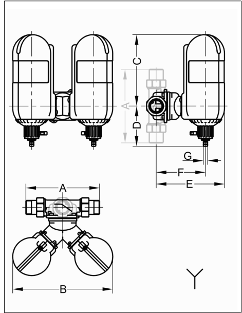
Fig. 12 : Cotes de montage JHF-T 1½" - 2"
