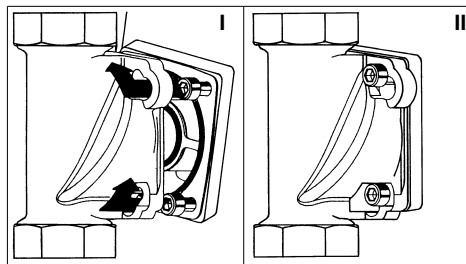
Fig. 4: Bride de montage rotative à baïonnette
