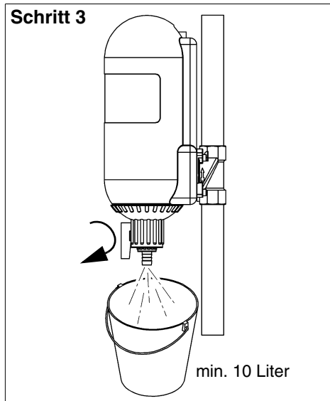
Abb. 8: Die Rückspülung wird gestartet, indem der Spülhahn aufgedreht wird. Ein Auffanggefäß mit mind. 10 Liter Volumen bereitstellen. Vorsicht Heißwasser, Verbrühungsgefahr!
