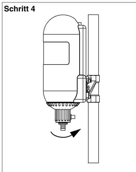
Abb. 9: Nach Beendigung der Rückspülung Spülhahn schließen und zurückdrehen. Ansonsten ist das Gerät nicht betriebsbereit!
