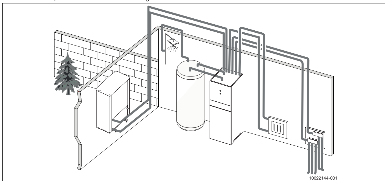
Bild 3 Wärmepumpe Compress 7001i AW, Inneneinheit AWMB mit integriertem Pufferspeicher und elektrischem Zuheizer, externer Warmwasserspeicher
