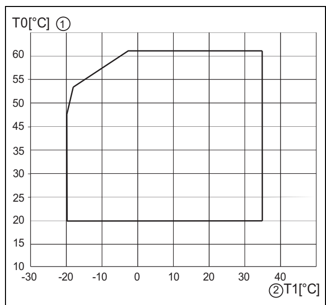
Bild 1 Wärmepumpe ohne Zuheizter
