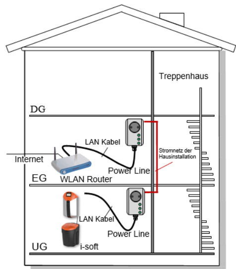
Power LAN Module am Router im EG und am i-soft im UG
