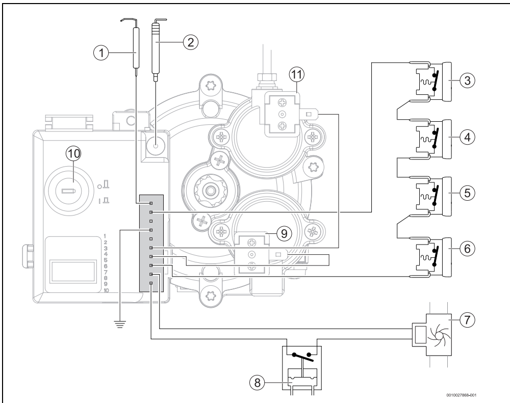
Bild 31 Schaltplan
