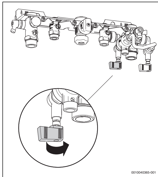
Bild 7 Füllleinrichtung öffnen
