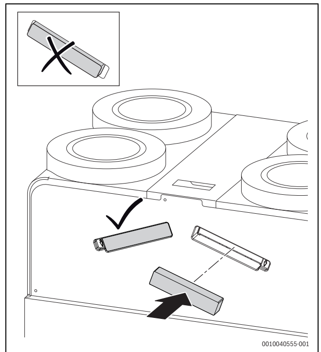
Bild 10 Filterabdeckung montieren
