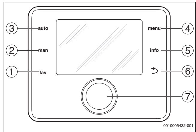
Bild 3 Bedienelemente
