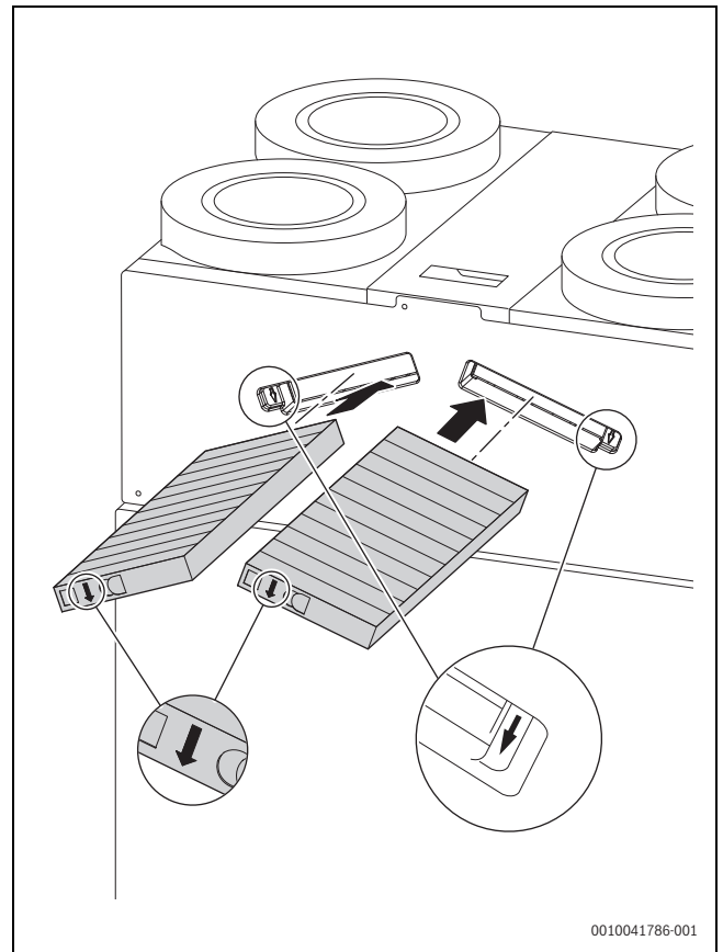
Bild 9 Filter einschieben
