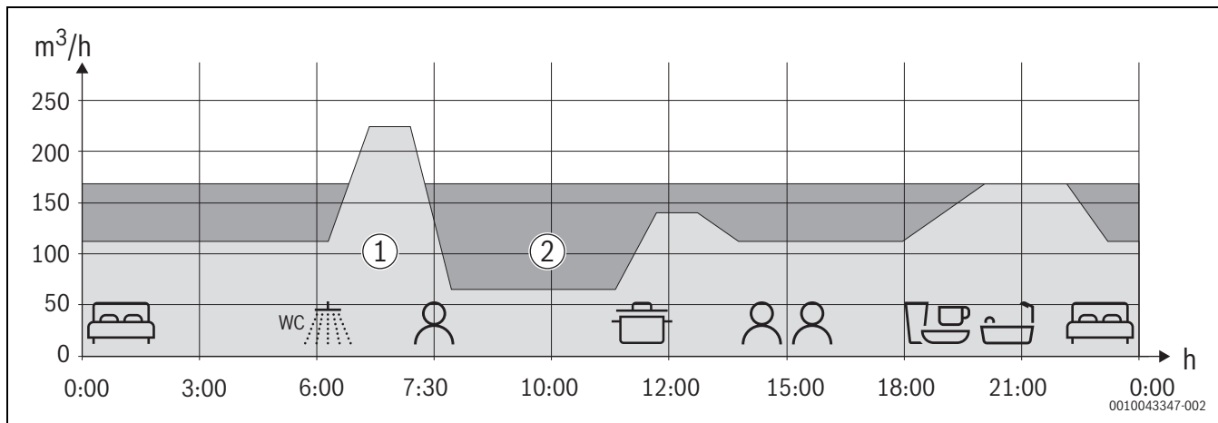
Bild 5 Beispielhafter Vergleich der bedarfsgeregelten/manuellen Lüftung
