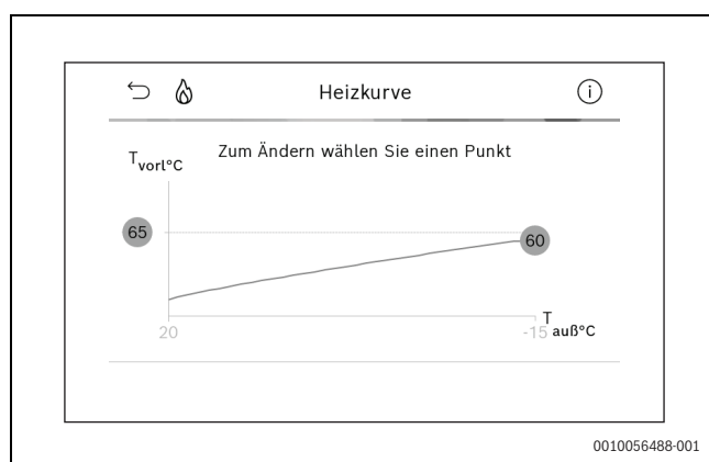
Bild 4 Außentemperaturgeführte Heizkurve mit den Einstellungen für Auslegungstemperatur und maximale Temperatur.
