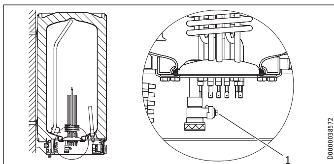
1 Zawór spustowy z przyłączem węża G 3/4
