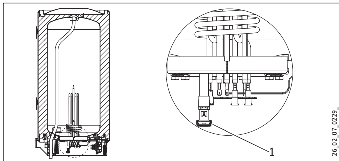
1 Capuchon de la vanne de vidange
