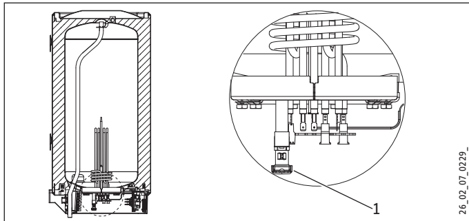
1 Kappe Entleerungsventil
