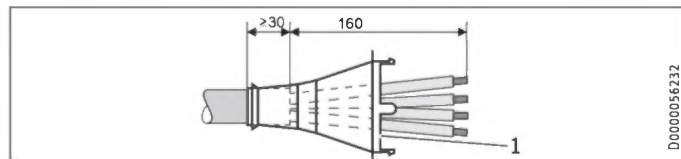
1 Kabeltülle
