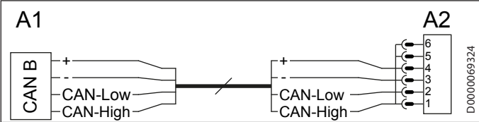
A1 Quadretto di comando WPM A2 Telecomando FET
