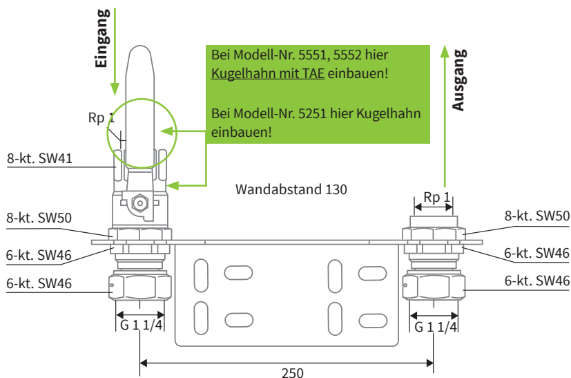
Abb. Modell-Nr. 5251
