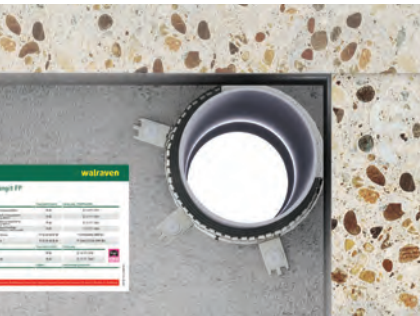
Besonders geeignet für Ecklösungen – 2/3 Umwicklung (abhängig von Rohrgruppe gemäß Verwendbarkeitsnachweis)
