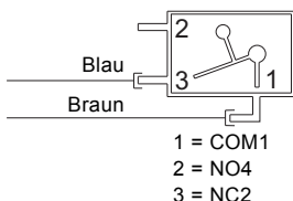
Abb. 1 Schaltbild
