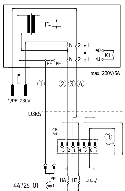
Schéma électrique
