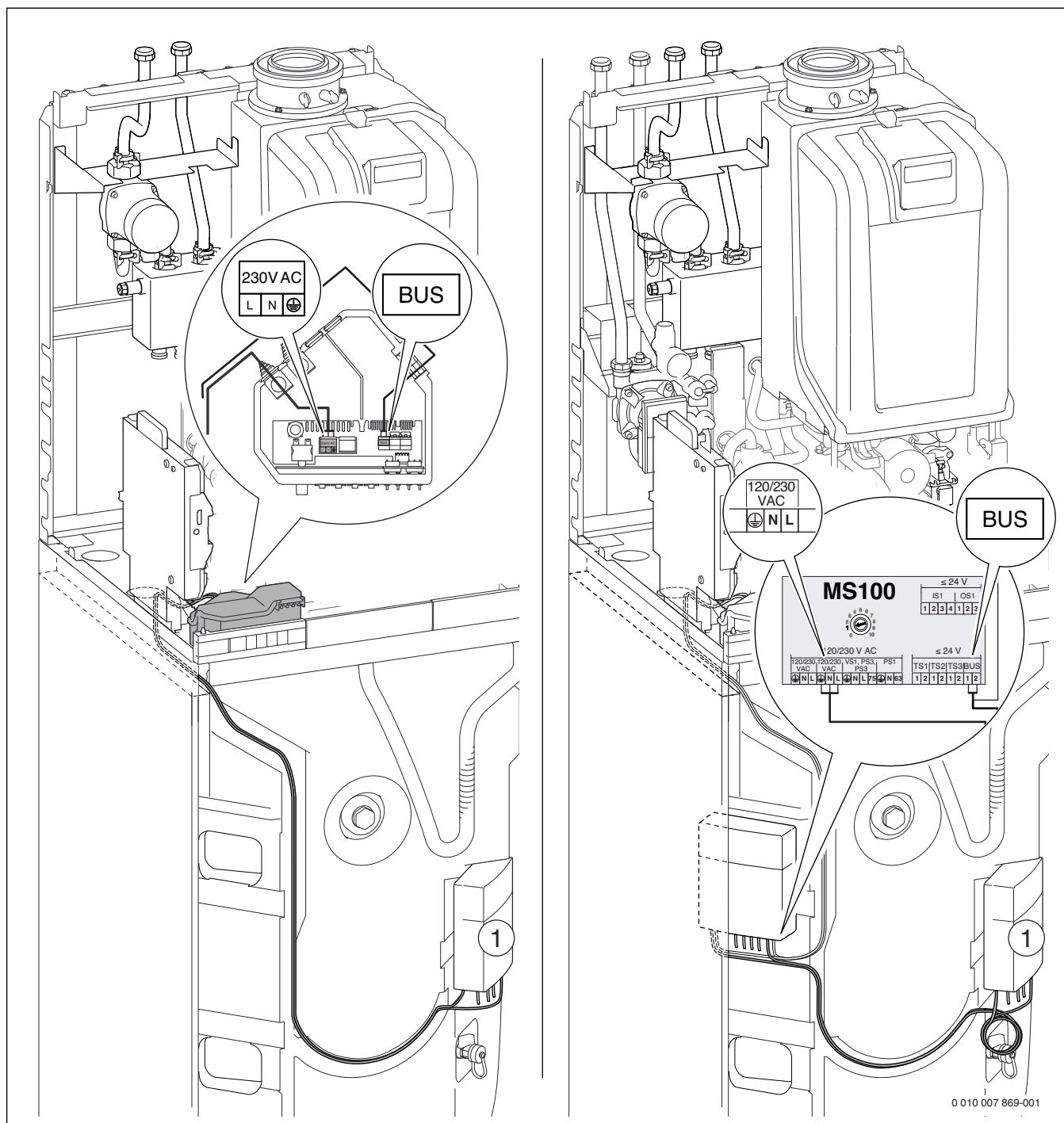
31 GB.192-..iT150-.. | GB.192-..iT150-..+CS22/Anschluss-Set solare Heizungsunterstützung SHU
