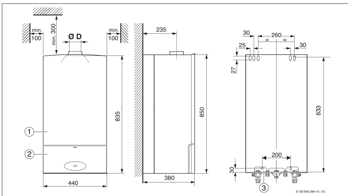
Bild 3 ZWR/ZSR 18/24... KE
