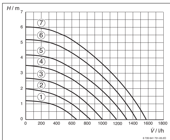
Bild 44 Pumpenkennlinien
