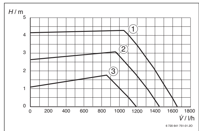
Bild 42 Konstantdruck
