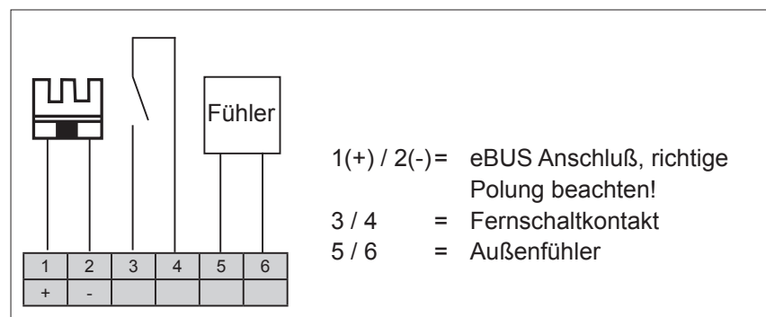
Abb. 4.8 Klemmenblockbelegung Wandschalter
