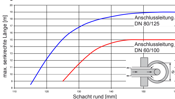
Abgasrohr DN 60
