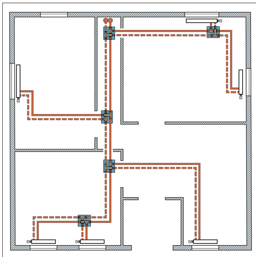
Abb. 2: Sanpress-Kreuzungs-T-Stück Anwendungsbeispiel Grundriss
