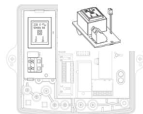
Netzmodul
