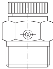
Entlüftungsautomat G 1/8", 1/4", 3/8"
