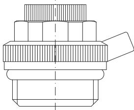
Entlüftungsautomat G 1/2" (selbstdichtend)
