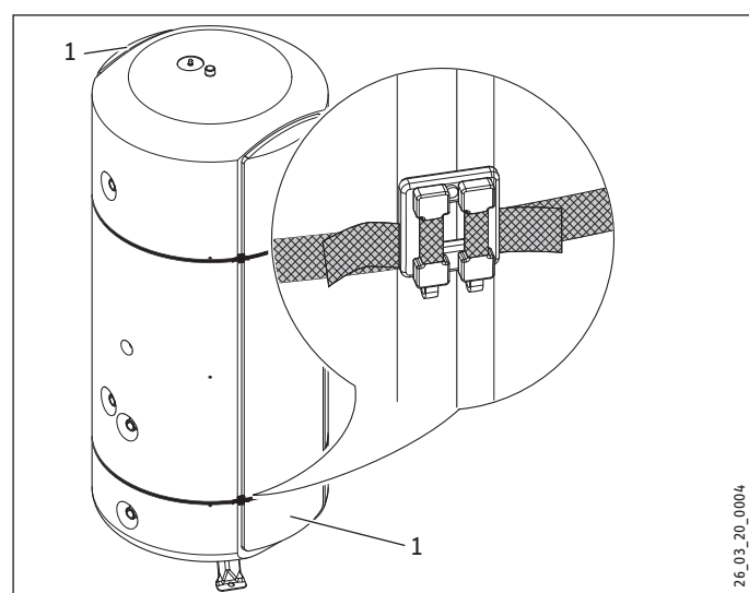
1 Segmento di isolamento termico laterale
