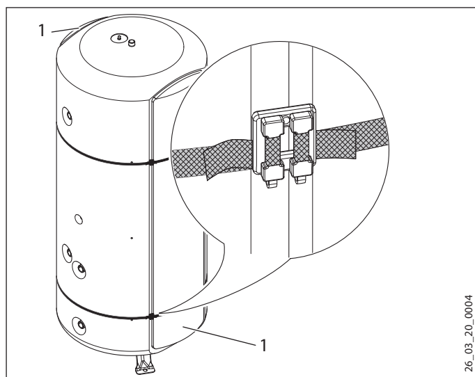
1 боковой теплоизолирующий элемент
