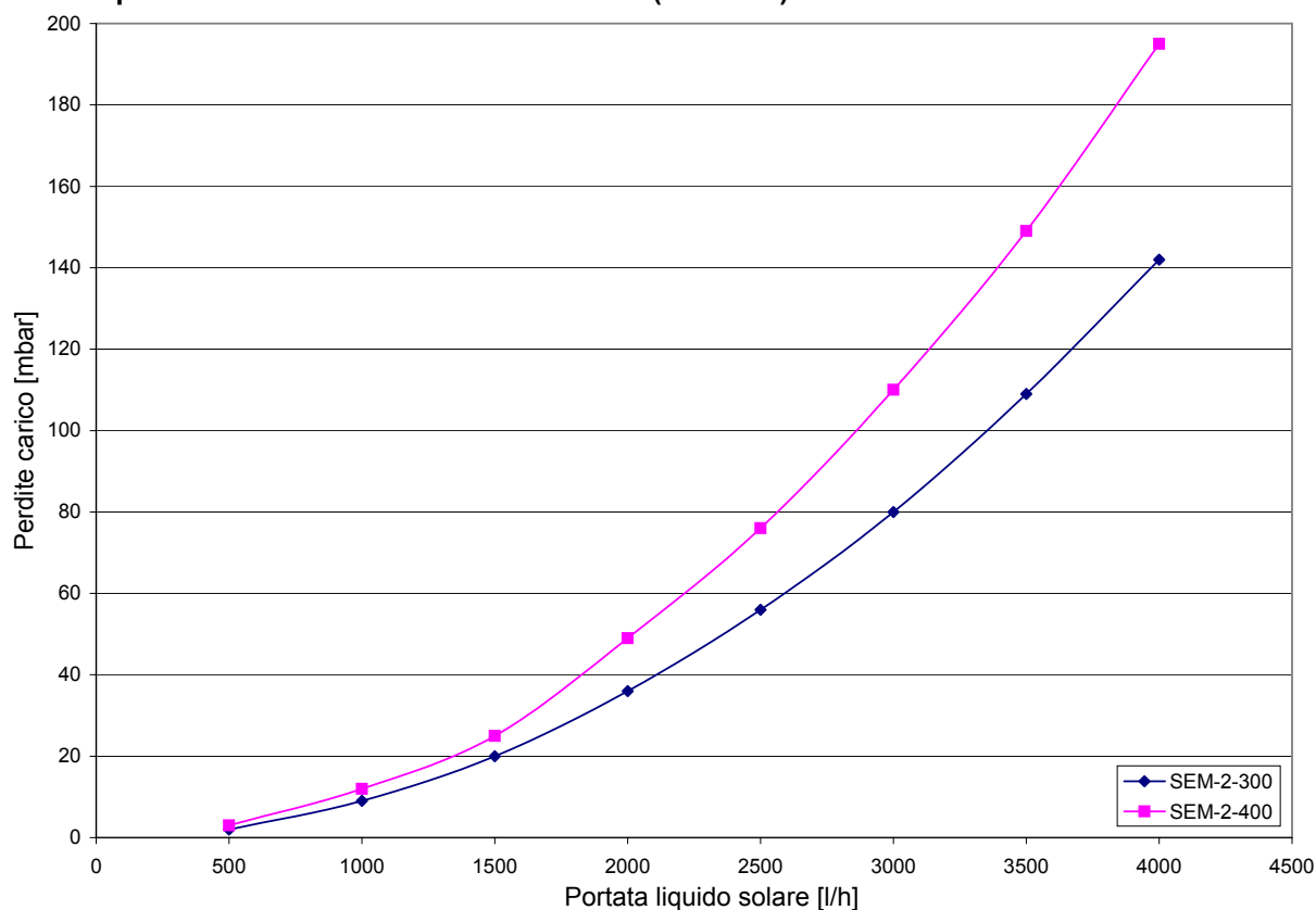
Perdite di carico serpentina di scambio termico lato solare (in basso)
