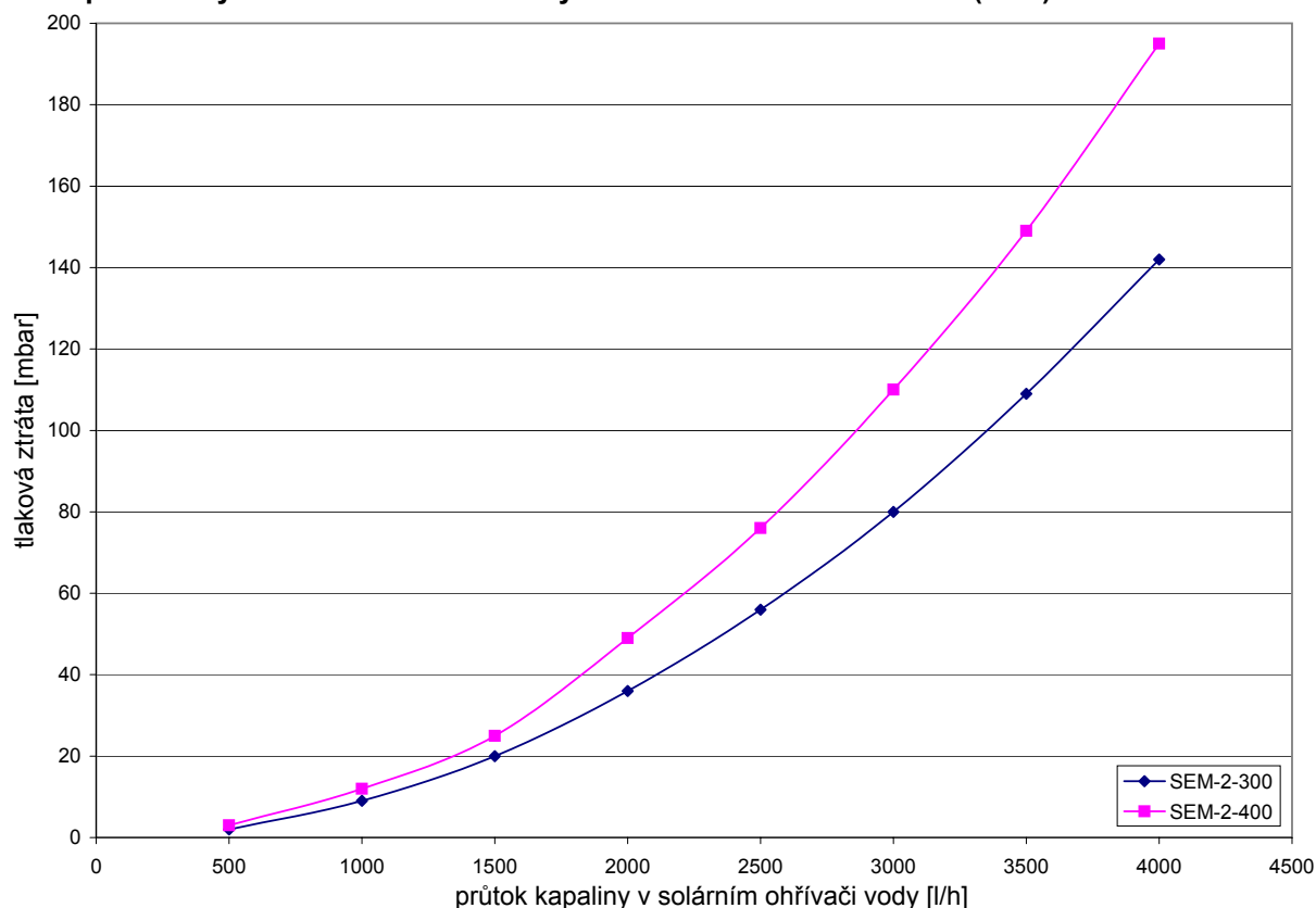
Tlaková ztráta otopné vložky solárního ohřívače vody na straně solárního zařízení (dole)
