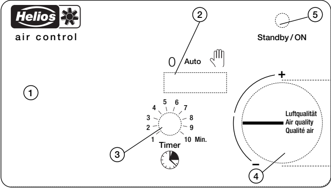
Bild 1: Gehäuseoberteil
