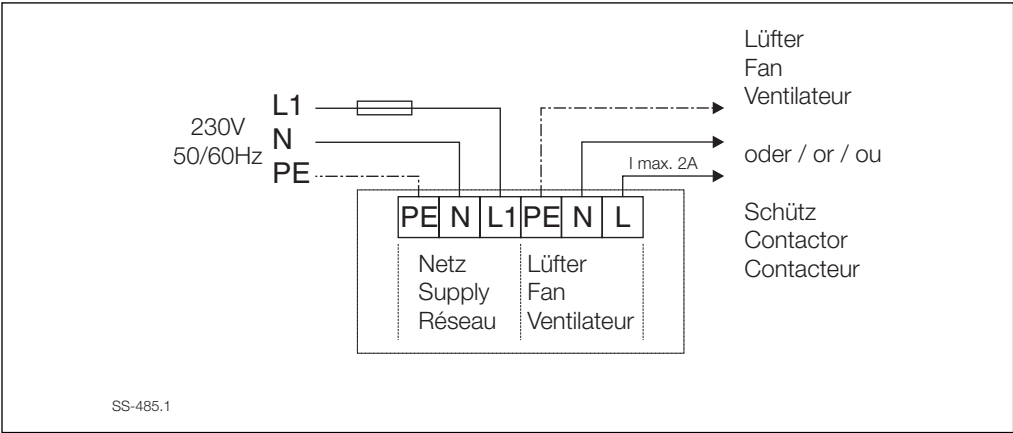
Bild 2: Anschlussplan
