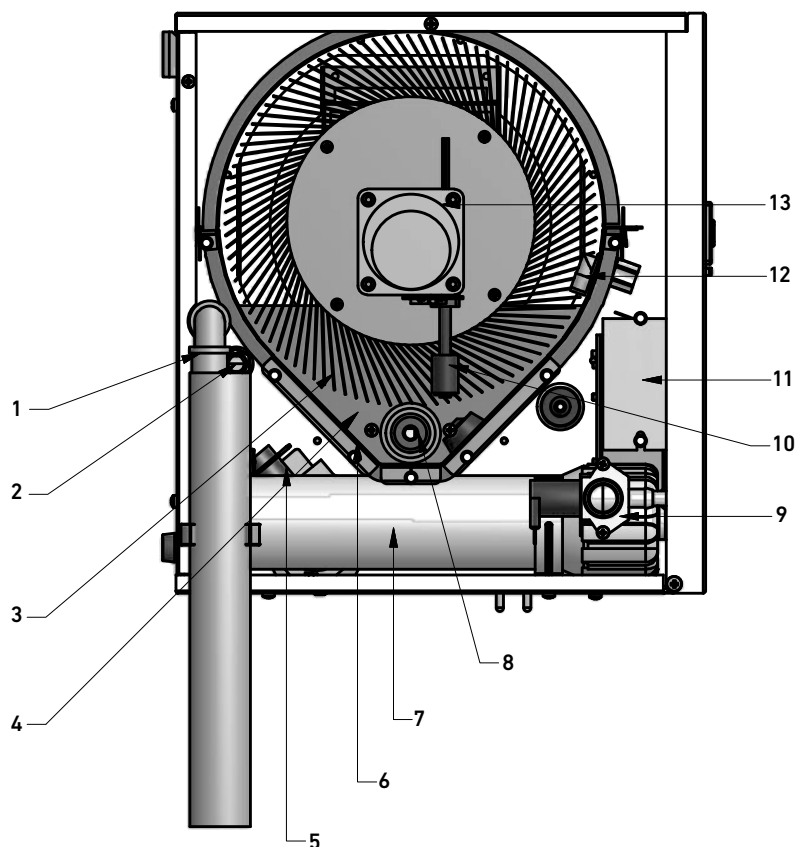
Abbildung: Funktionsansicht
