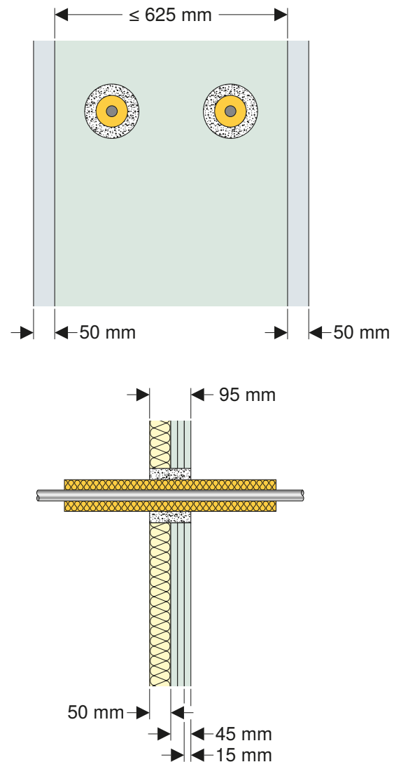
Abbildung 2: Dimensionierung Schachtwände
